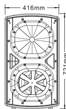
正视图
