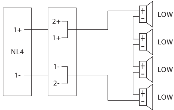
1 + 1- INPUT
